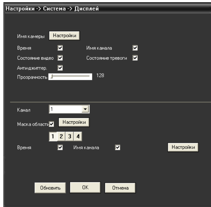
Рис. 3.46 Дисплей.
