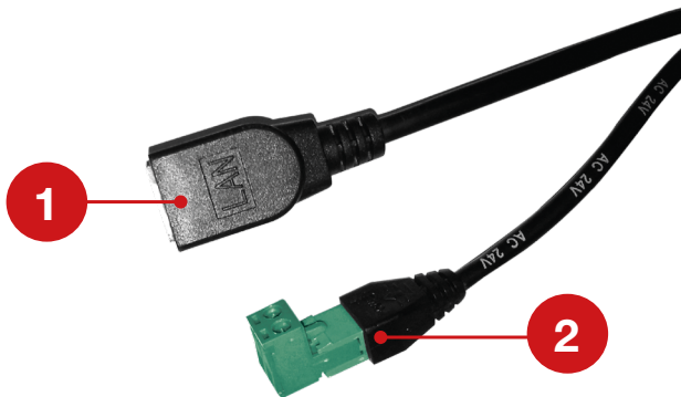
Рис.2.14 Разъемы камеры.
